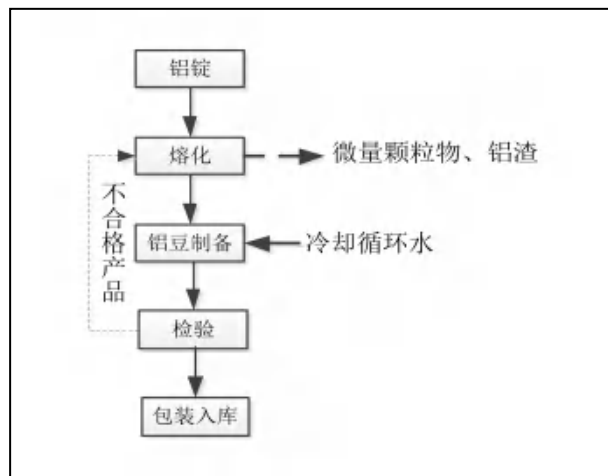
图 2-3 铝豆生产工艺流程及产污环节图
