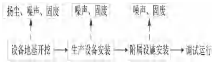
图 2-2 项目施工期工艺流程及产污环节图
