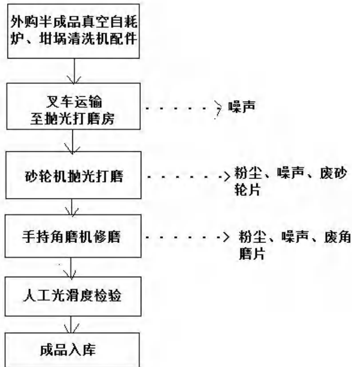
图 2-3 项目生产流程图
